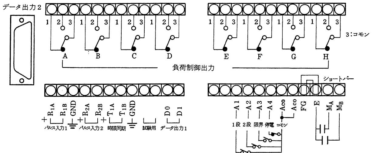
図5 端子配列図
