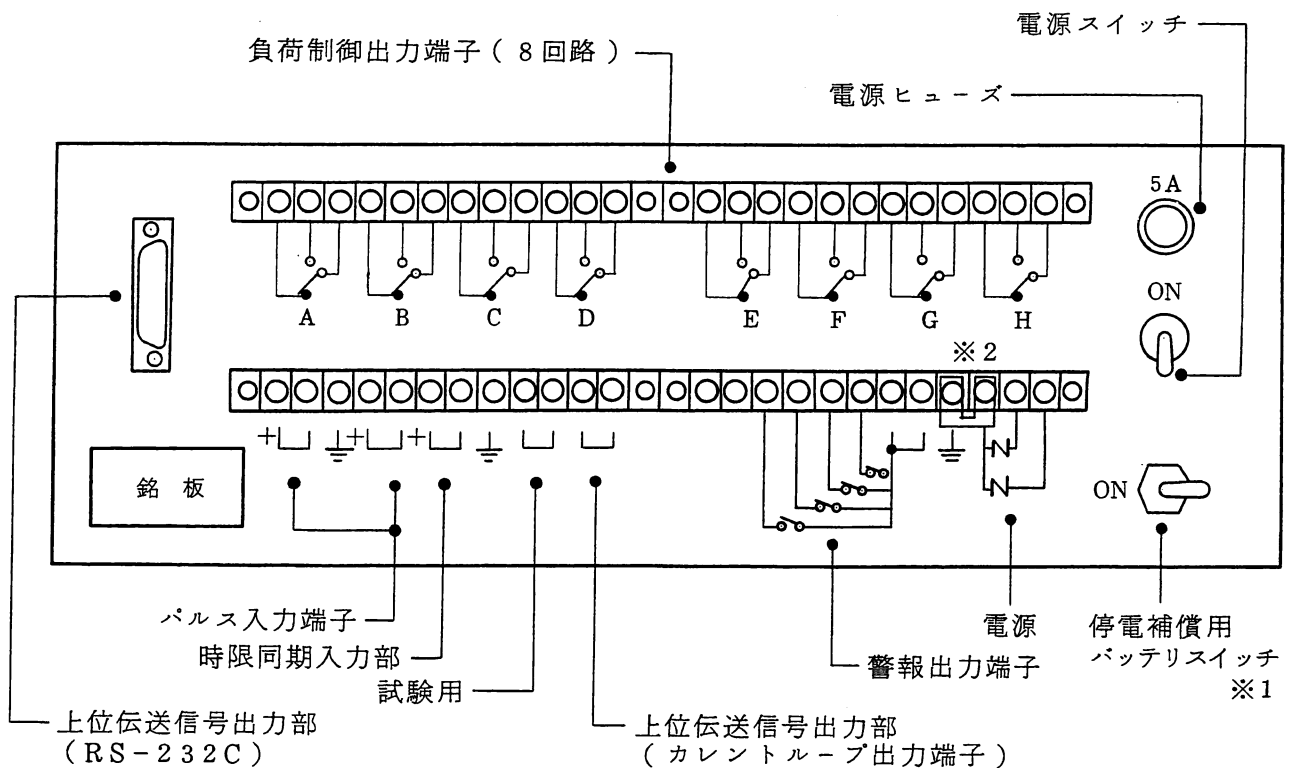
図2 リアパネル
