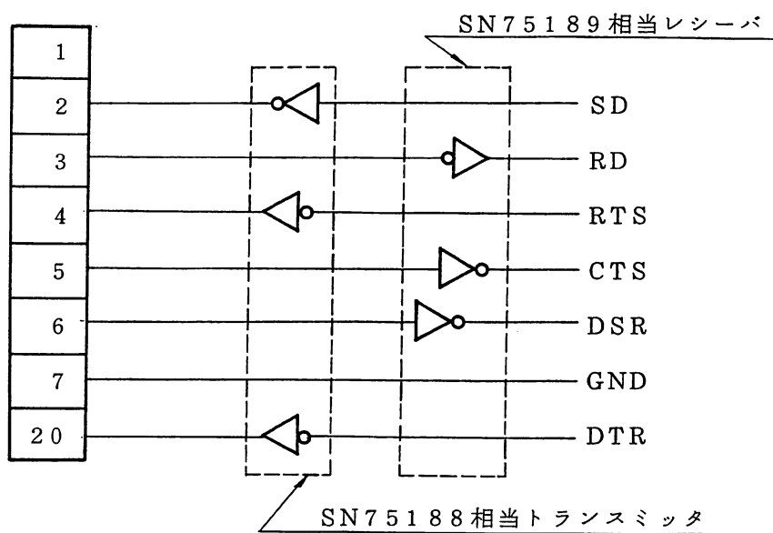
図6 データ出力2 コネクタ内部接続図
