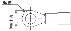
図 絶縁被覆付圧着端子
