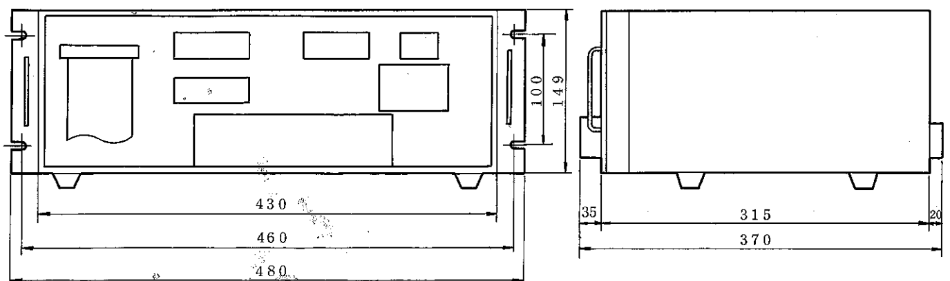
(外形寸法)
