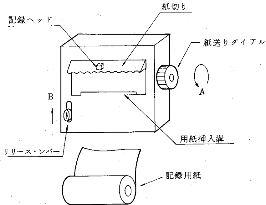
図9 プリンタと記録用紙
