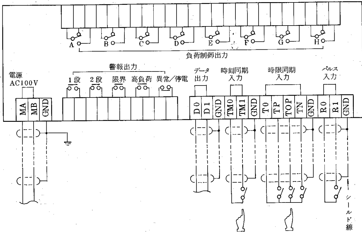
図 3 端子配列図
