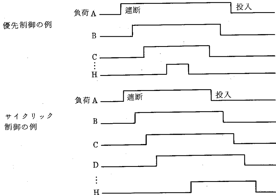
図21 負荷制御動作
