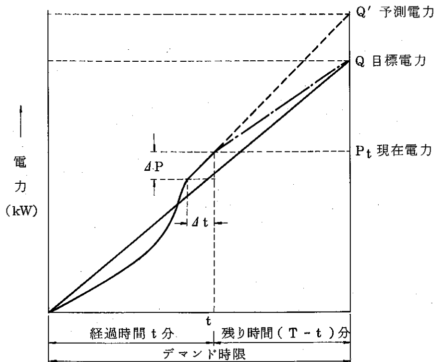
図 20 デマンド値とデマンド時限の関係動作図
