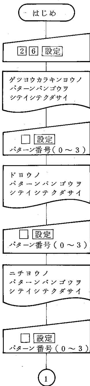
図 19 時間帯指定 2 設定フローチャート
