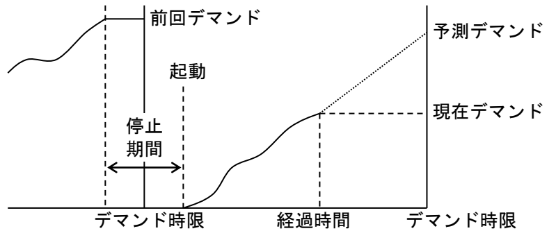
図 11-3 デマンド時限を越える期間の停止
