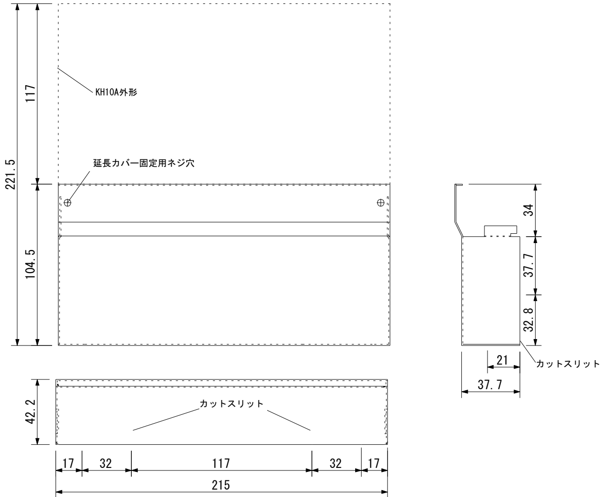
延長カバー使用時の取付寸法
