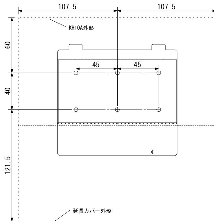
延長カバー使用時の取付寸法
